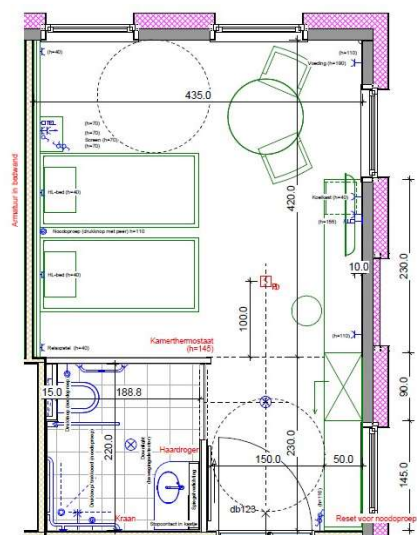
Type 2 - 2 persoonskamer - 23m 2
